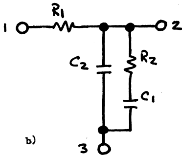
Fig. 3: RIAA NETWORKS ( T_1=3180\mu s , T_2=318\mu s , T_3=75\mu s )
